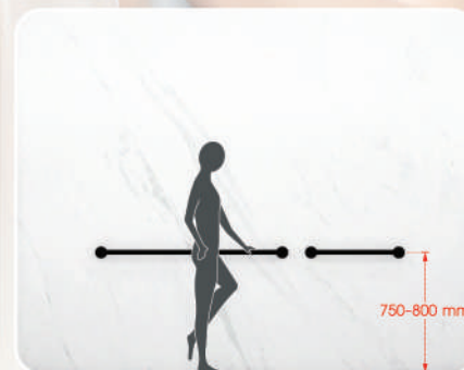
รูปแบบการติดตั้งบนพื้นที่ต่างระดับ และพื้นราบ
